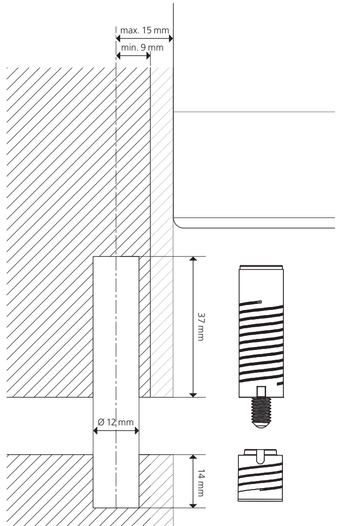
Invis Mx2 Eindrehmutter 14 mm Invis Mx2 stud 14 mm
