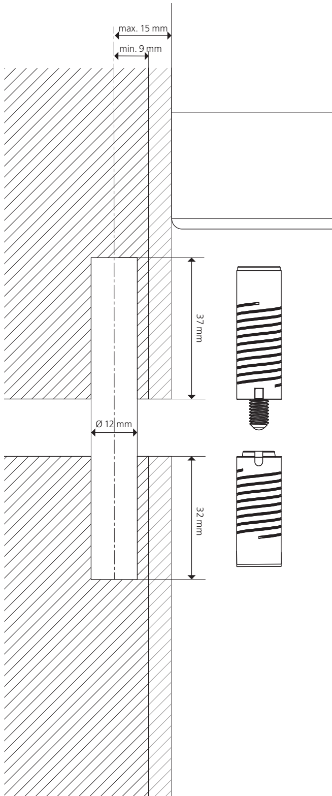
Invis Mx2 Eindrehmutter 30 mm / Invis Mx2 stud 30 mm
